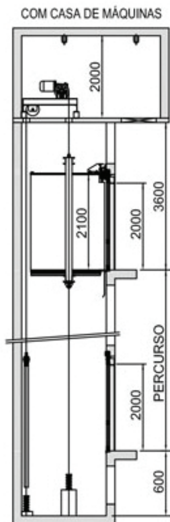
CORTE LATERAL
