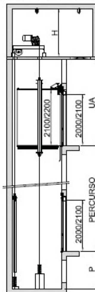
CASA DE MÁQUINAS C/ UM NÍVEL
