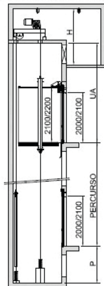
CASA DE MÁQUINAS C/ DOIS NÍVEIS
