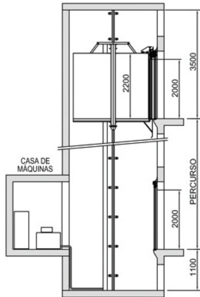
CORTE LATERAL
