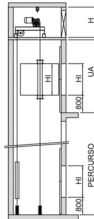
CORTE LATERAL
