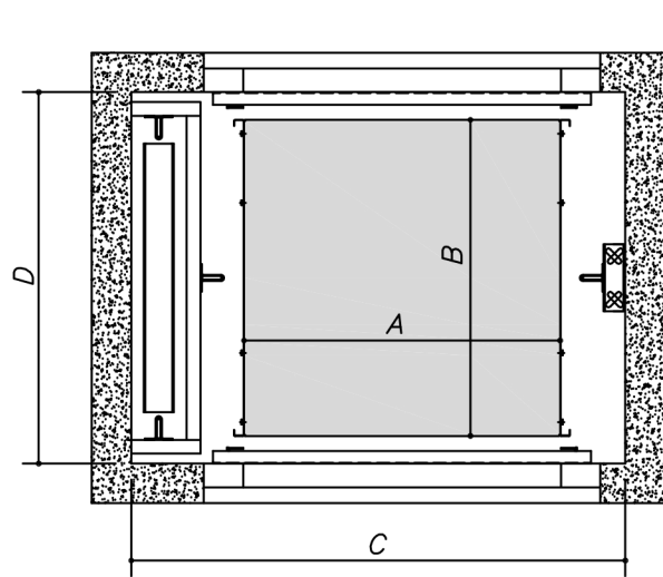
ENTRADAS OPOSTAS
